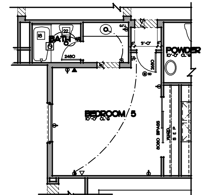
OPTIONAL BEDROOM 5 W/BATH IN LIEU OF HOME THEATER
