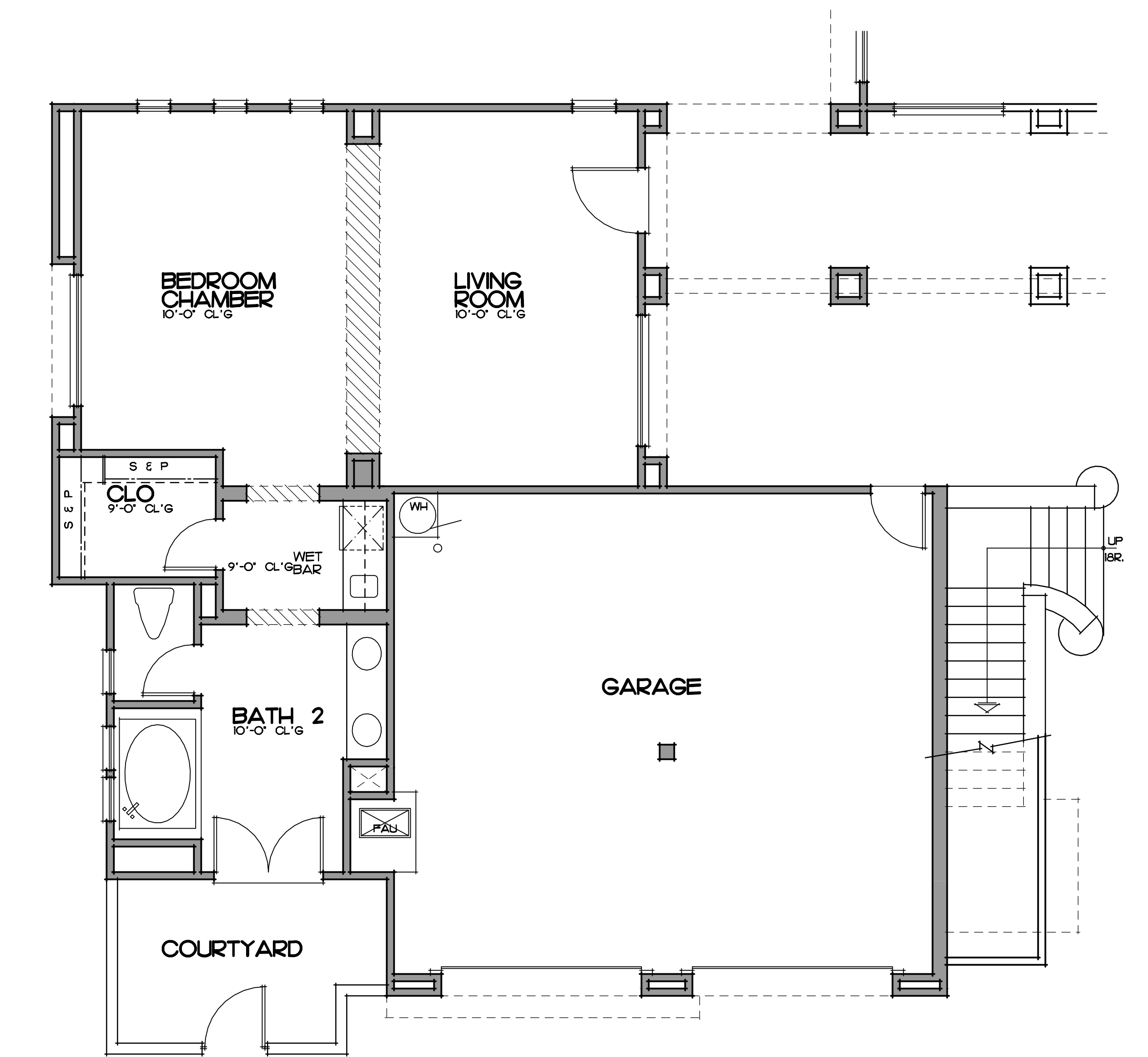
OPTIONAL CASITA PLAN 'A' SCALE: 1/4" = 1'-0"
