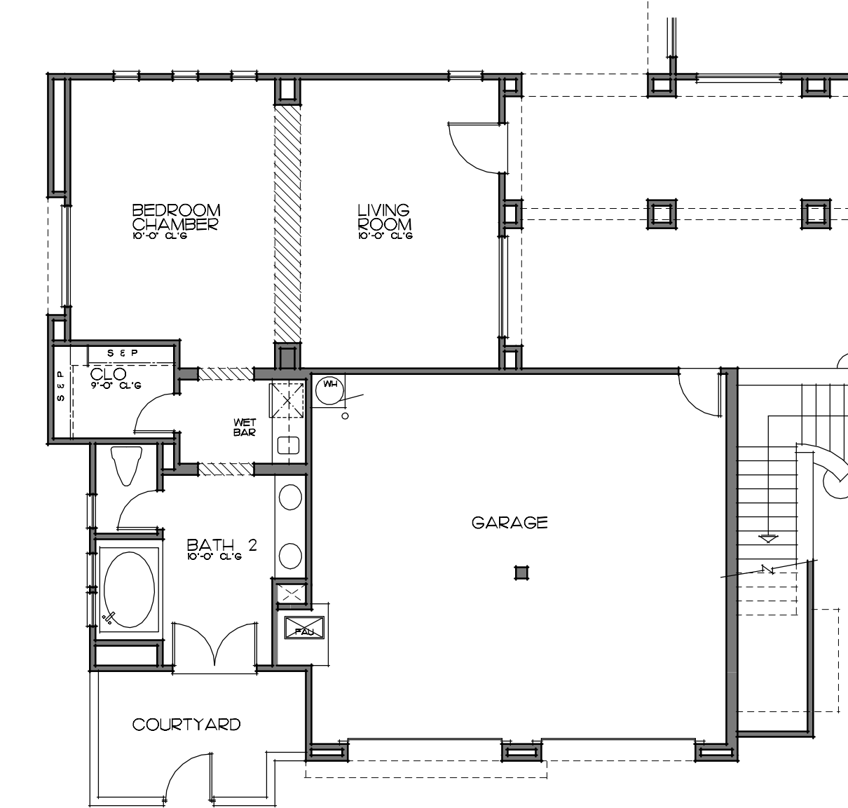
OPTIONAL CASITA PLAN 'A' SCALE: 1/4" = 1'-0"
