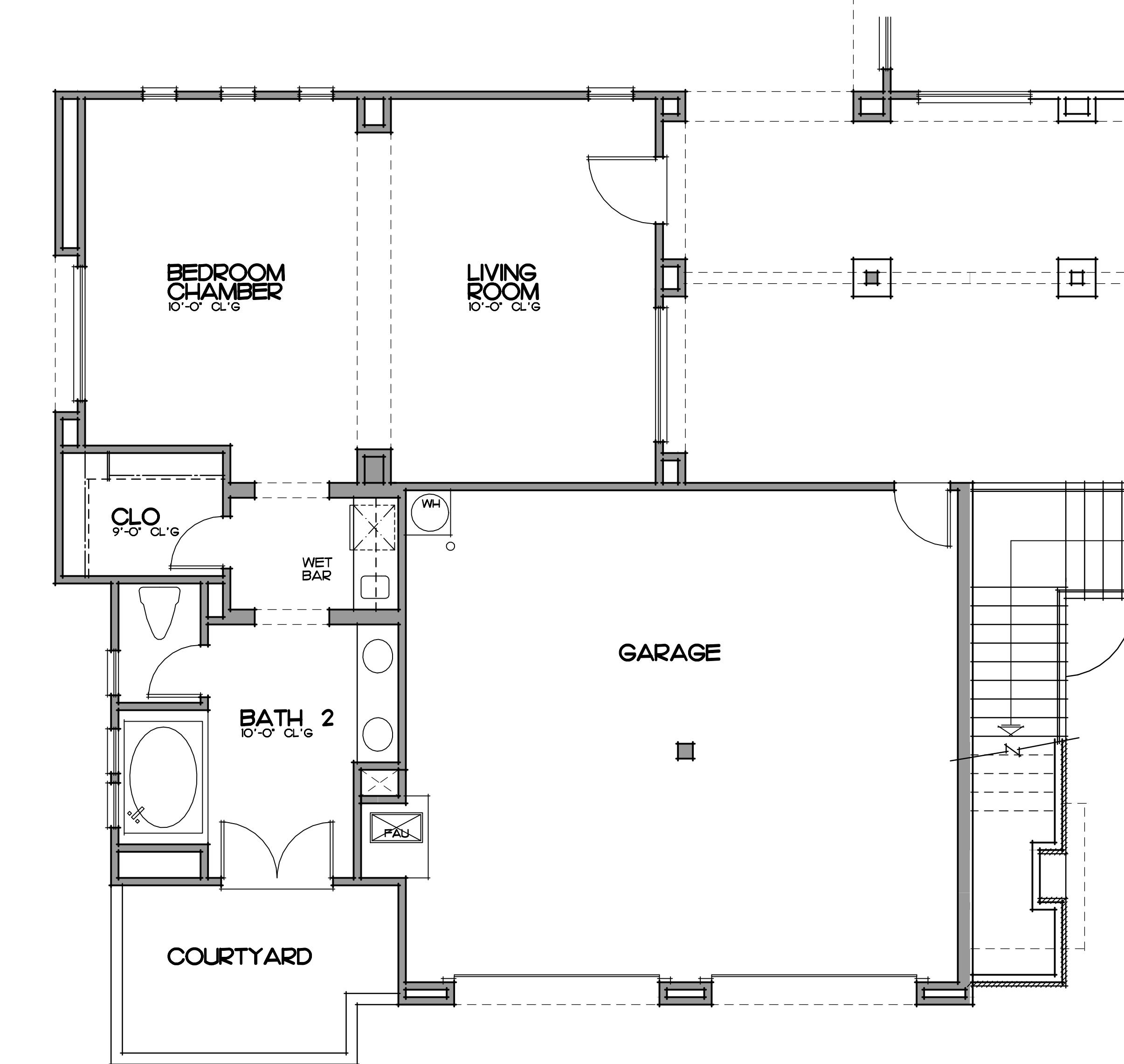
OPTIONAL CASITA PLAN 'B' SCALE: 1/4" = 1'-0"
