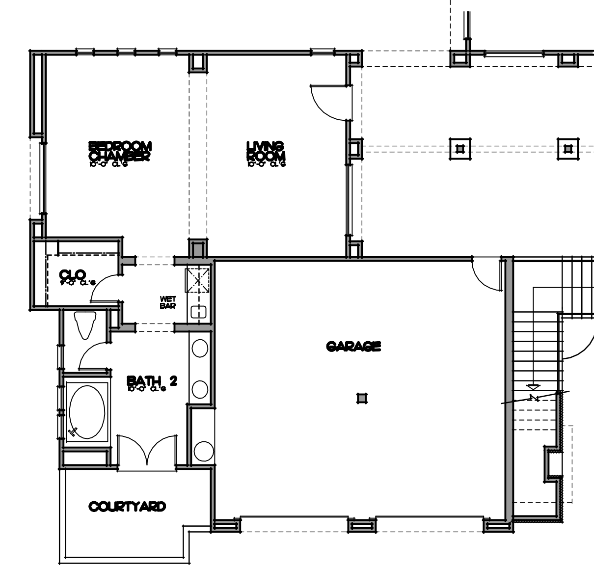
OPTIONAL CASITA PLAN 'B' SCALE: 1/4" = 1'-0"
