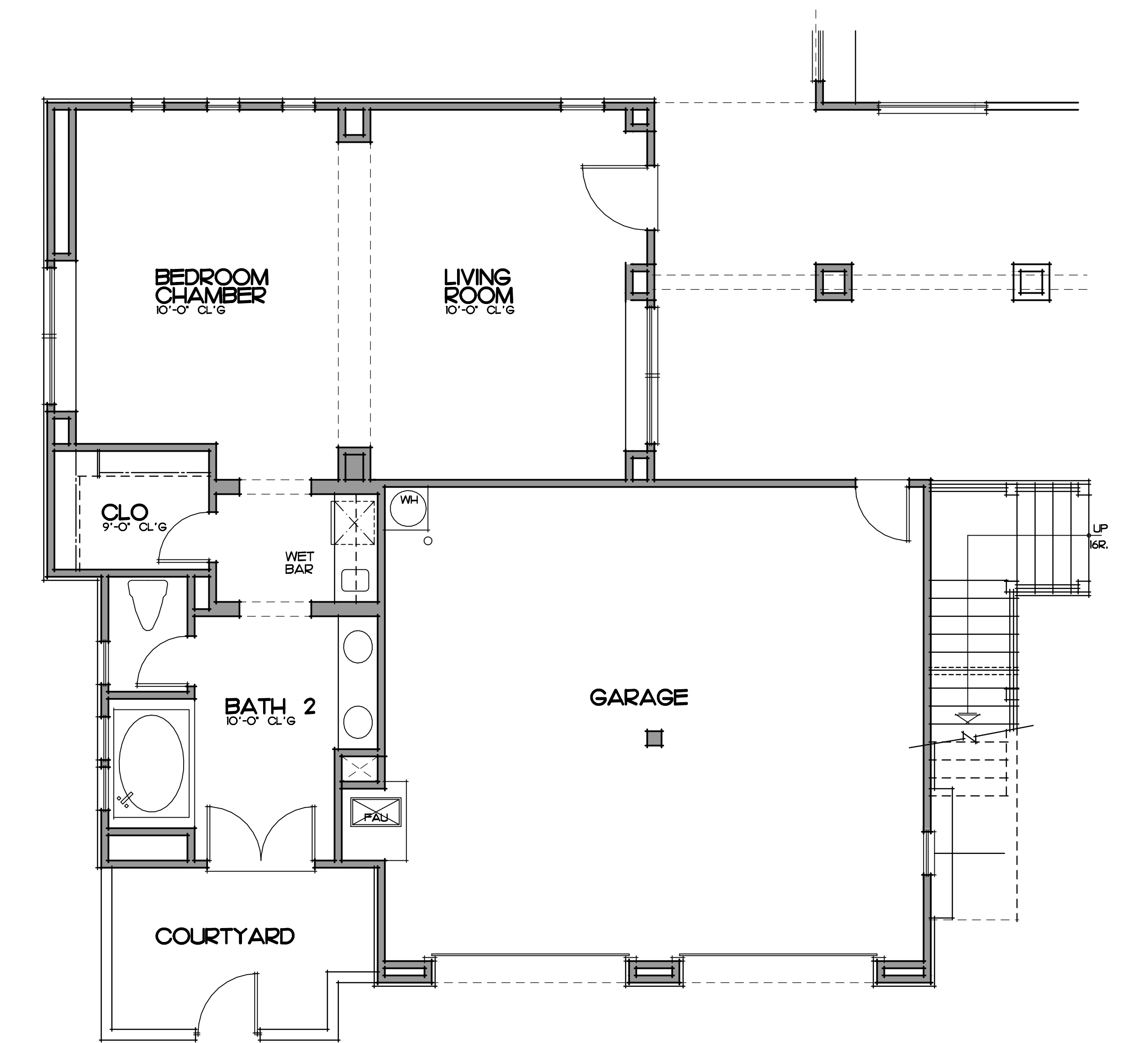
OPTIONAL CASITA PLAN 'C' SCALE: 1/4" = 1'-0"
