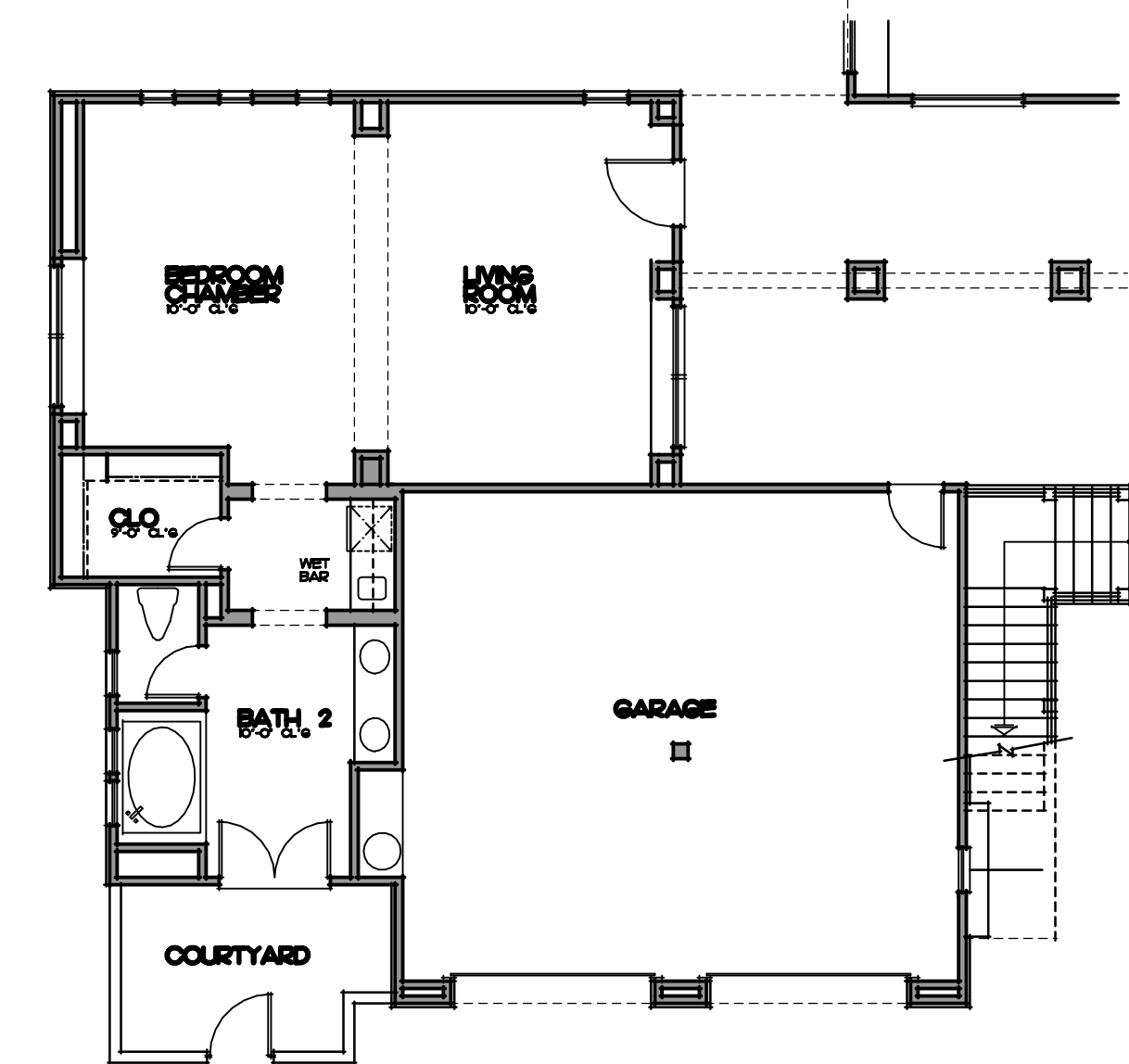
OPTIONAL CASITA PLAN 'C' SCALE: 1/8" = 1'-0"
