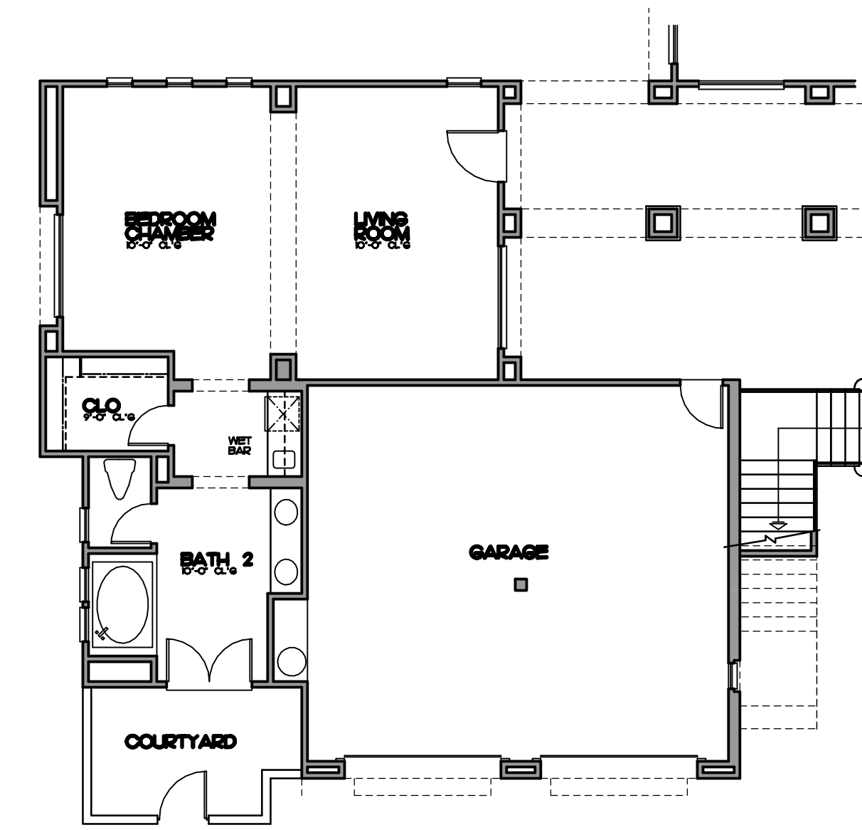
OPTIONAL CASITA PLAN 'D' SCALE: 1/4" = 1'-0"
